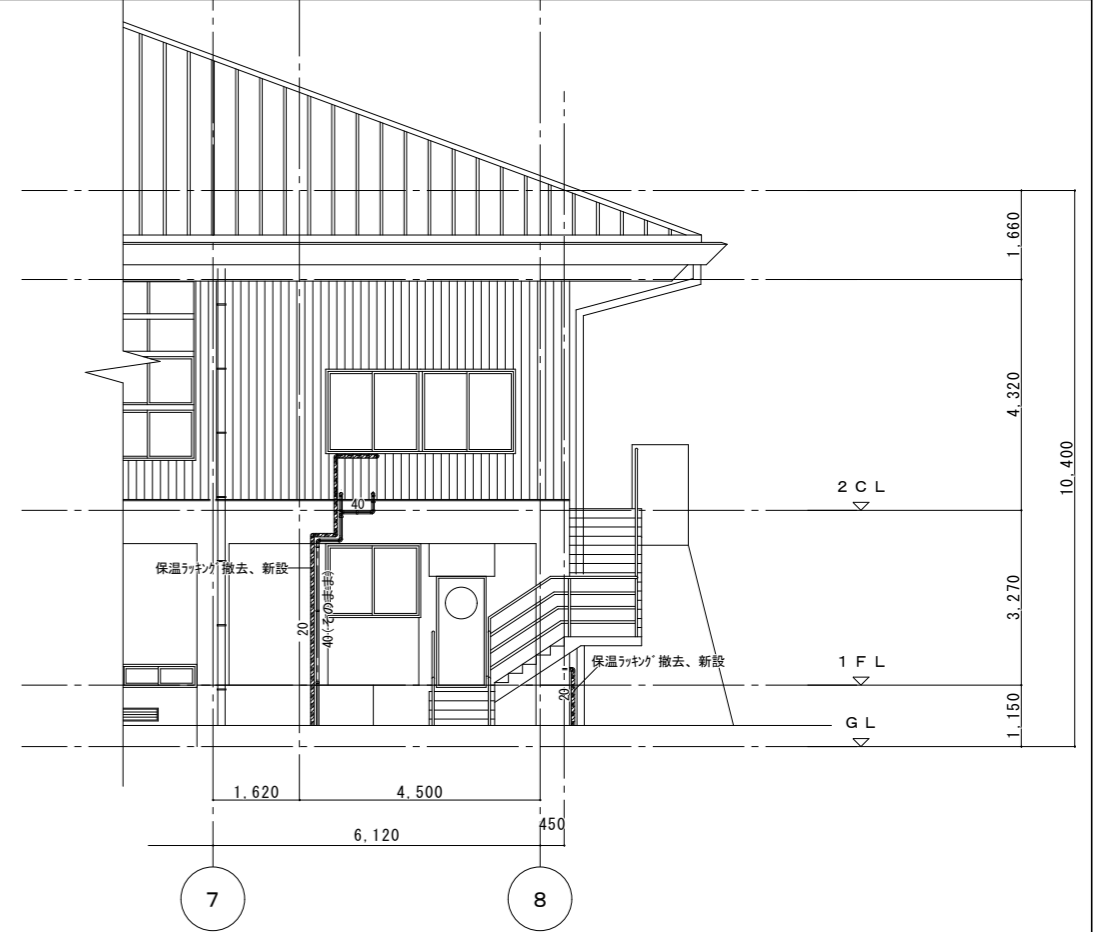
給水管保温ラッキングやり替え参考図
